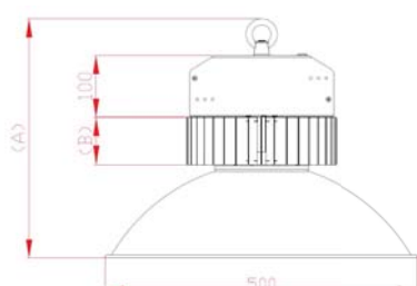
rozměry modelů HB-50 až HB-200
