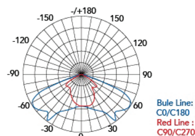
vyzařovací charakteristika
