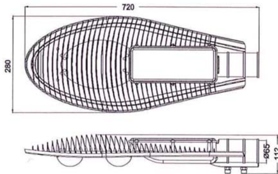
rozměry SLCD2
