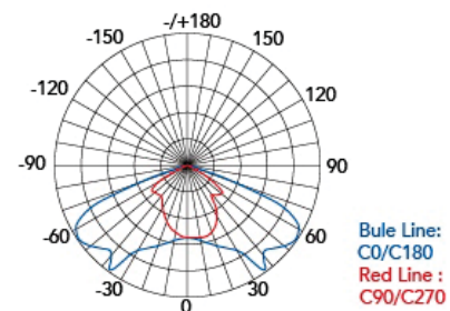
vyzařovací charakteristika
